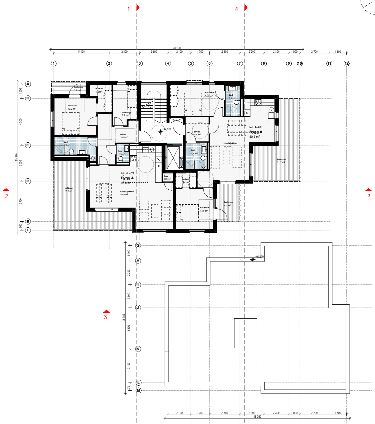
4. etasje
