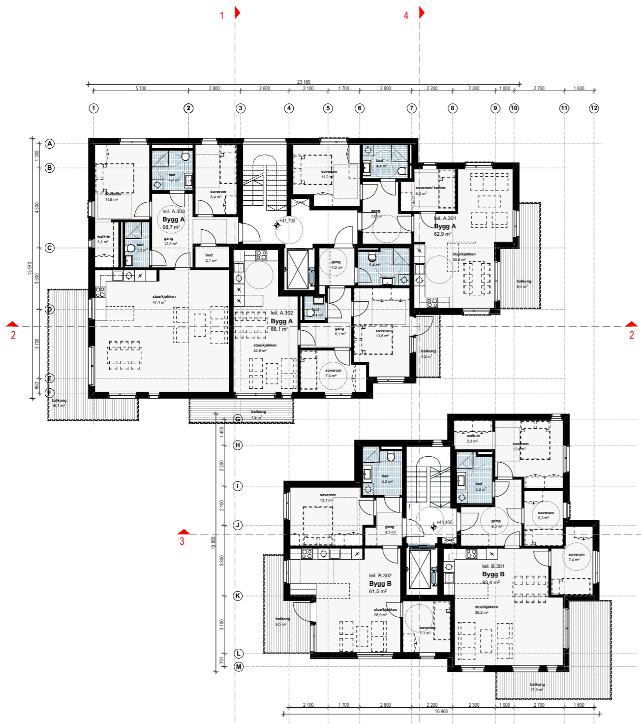
3. etasje
