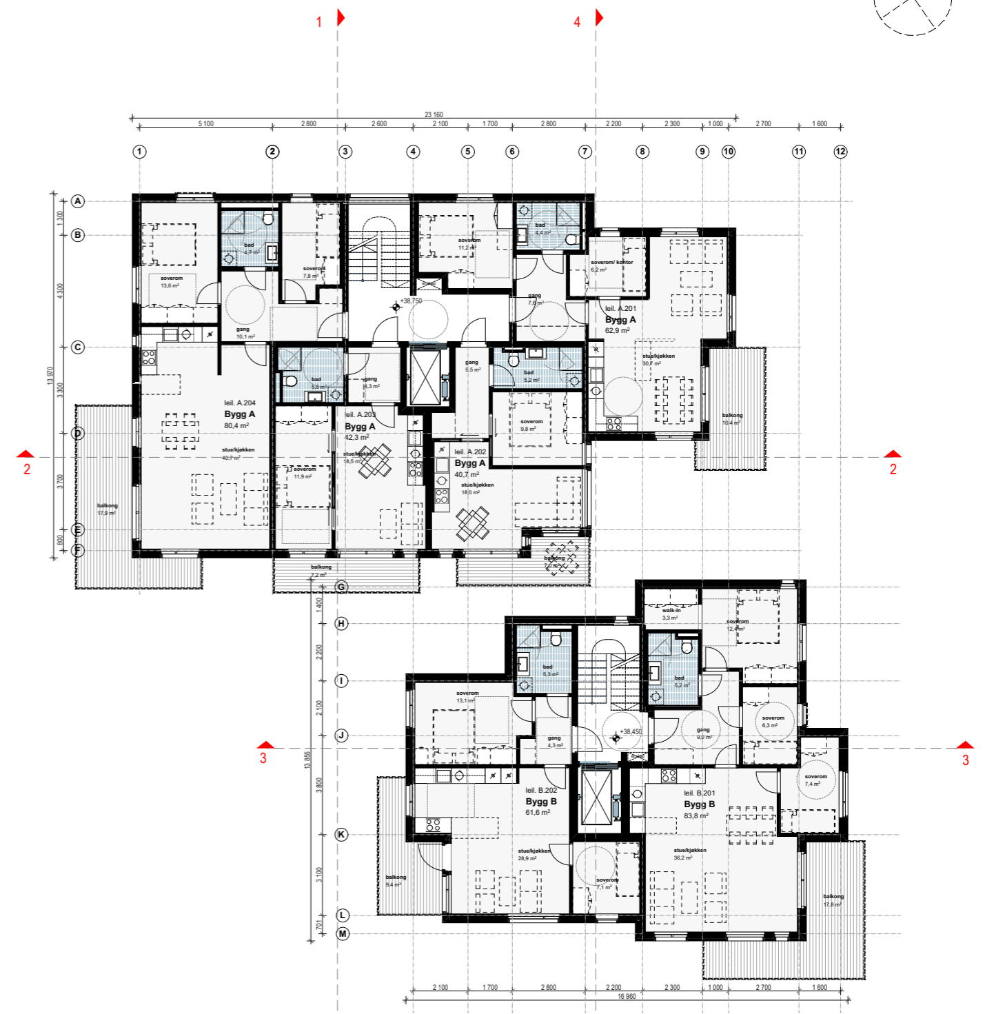
2. etasje
